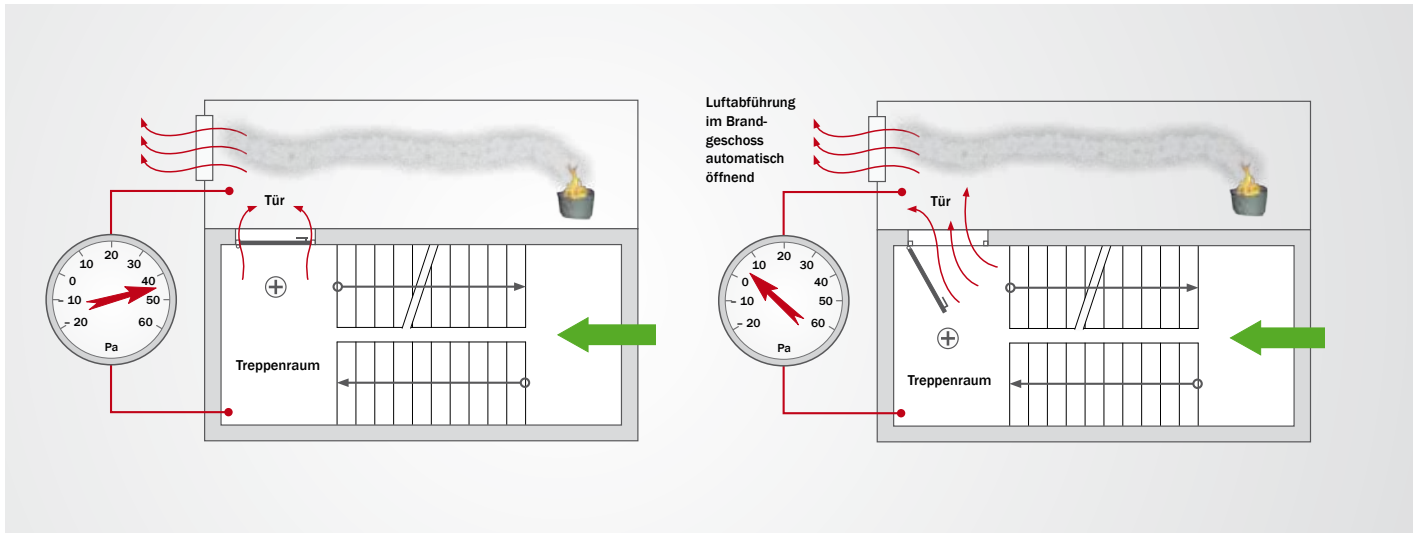
Abb. 2: Differenzdruck an der zu schützenden Tür
